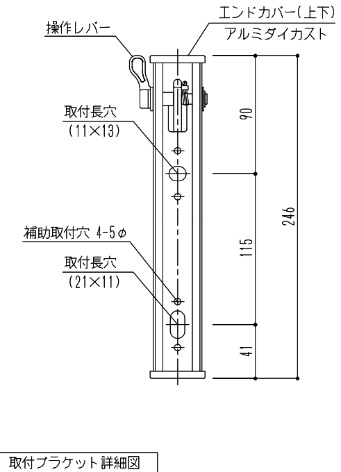
取付ブラケット詳細図
